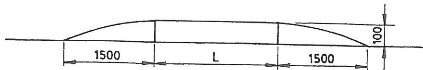
c. Próg płytowy typu 1A 2
